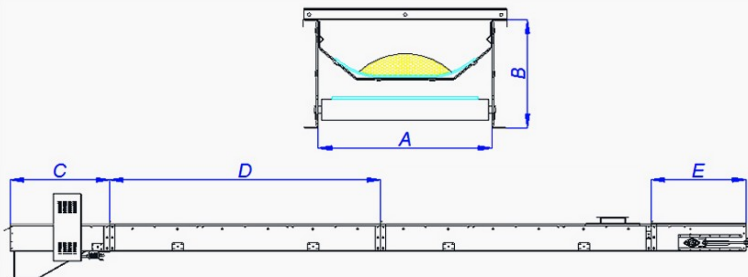
Размеры конвейера модели BKV
